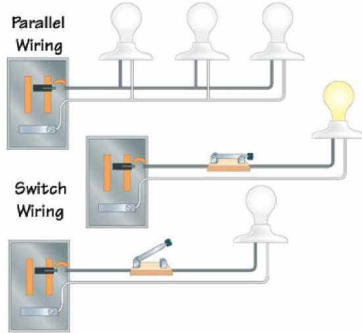
चित्र 2.1.5 समानांतर और स्विच वायरिंग
