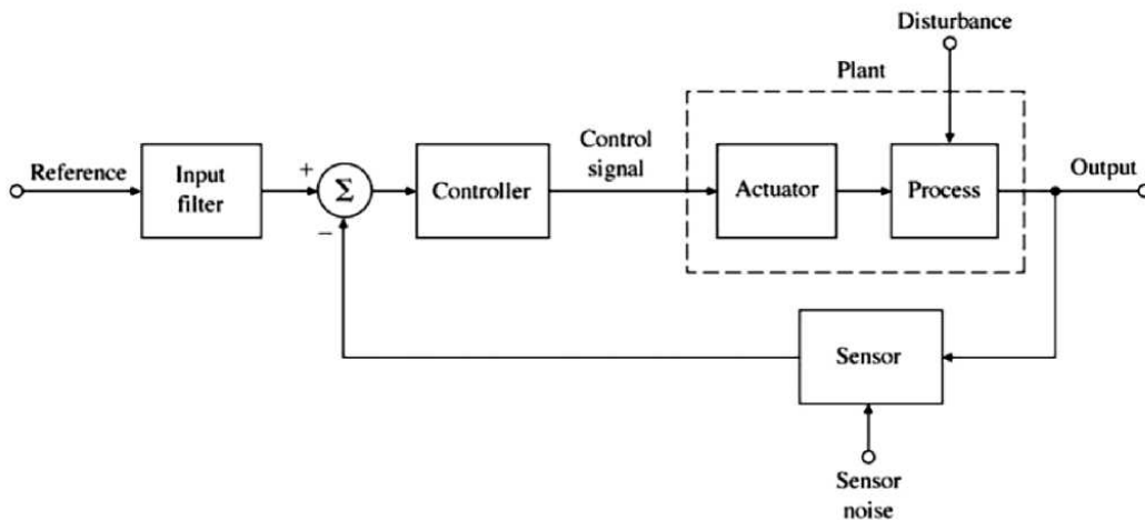
चित्र 1.2.1.5 (ए) ब्लॉक आरेख
