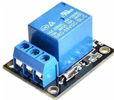
चित्र 2.1.11 रिले
