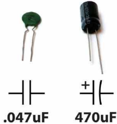
चित्र 1.2.1 (एफ) कैपेसिटर
