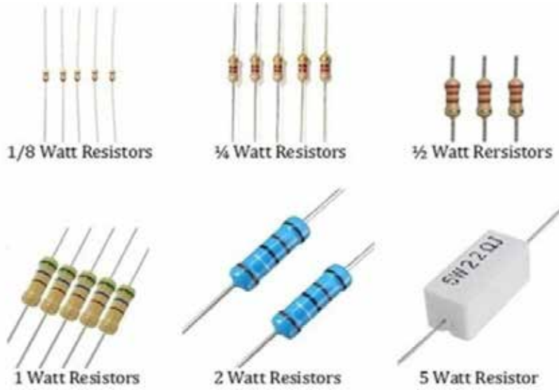
चित्र 2.1.1 प्रतिरोधों
