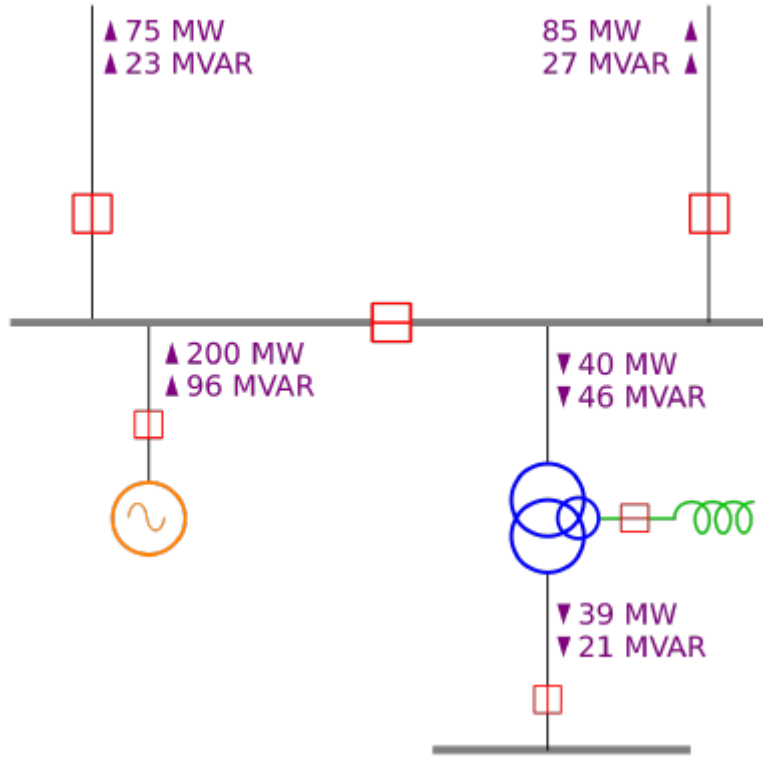
चित्र। 2.1.5 (सी) रेखा आरेख
