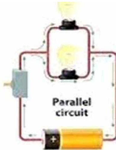
चित्र 2.1.6 समानांतर परिपथ
