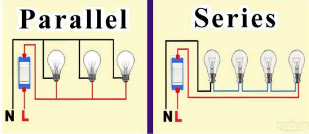
चित्र 2.1.5 समानांतर और श्रृंखला वायरिंग
